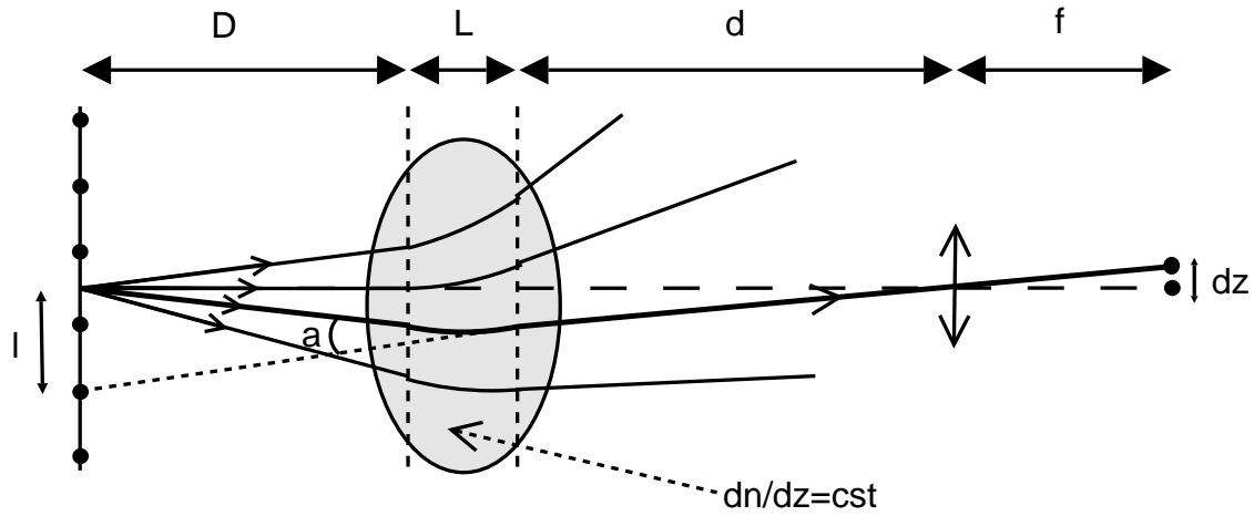
FIG. 1 – Tracé de rayons en schlieren synthétique. Le chemin réel (en gras) diffère du chemin en l'absence de gradient d'indice (en tirets), ce qui amène à une translation dz dans le plan image.
