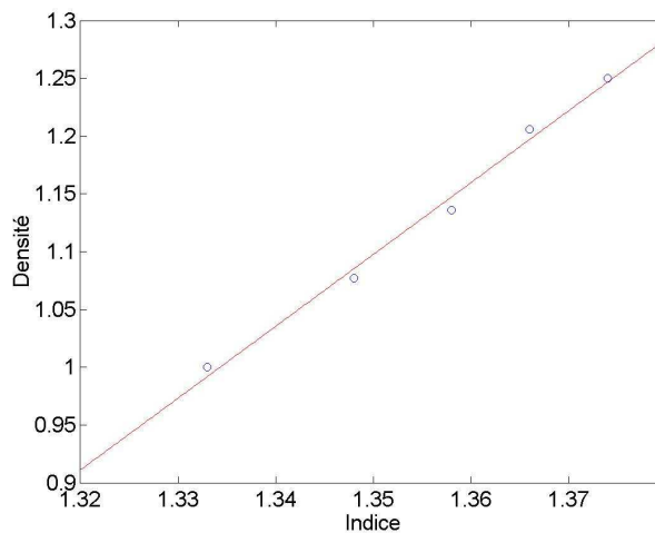
FIG. 2 – Relation linéaire entre la densité des solutions de NaNO_3 et leur indice optique.
