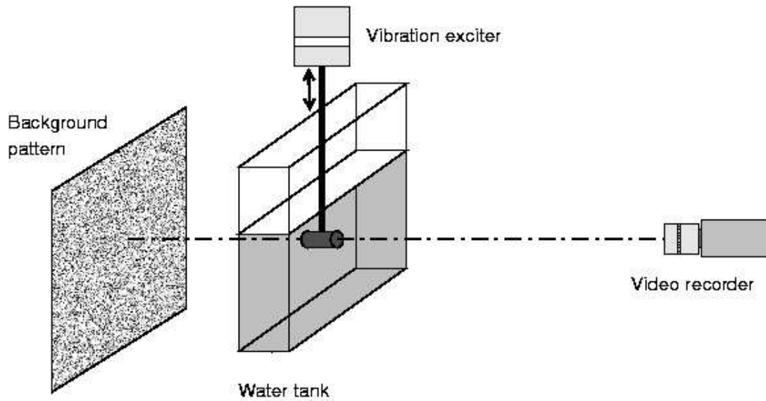
FIG. 3 – Dispositif expérimental.
