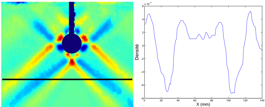
FIG. 5 – Croix de St André émise par un cylindre de rayon 1,5cm (visible au centre) oscillant à 0.15Hz avec une amplitude de 1.5mm. A droite, perturbation de densité selon la coupe horizontale représentée par le trait noir.
